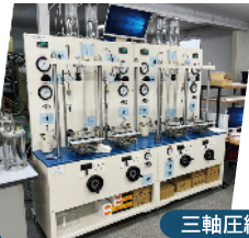
三軸圧縮試験
